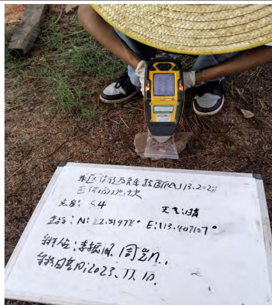
S4--XRF
